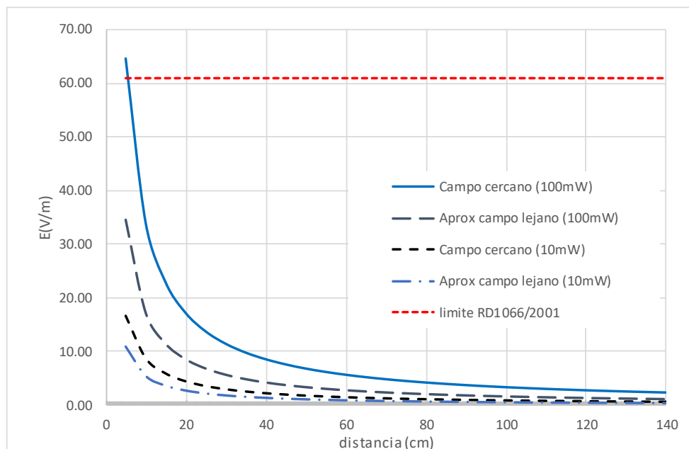
Figura 4. Variación del nivel de campo eléctrico (rms) con la distancia para la transmisión en la banda de 2,4 GHz con un dipolo corto y diferentes valores de PIRE, en espacio libre.
