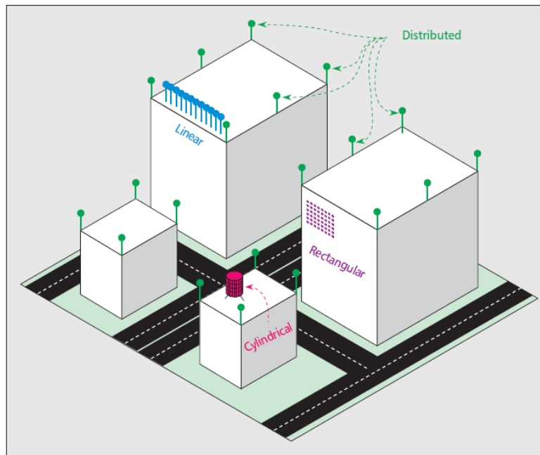
Figura 2 Configuración MIMO masivo lineal (azul), rectangular (violeta), cilíndrico (magenta) o distribuido (verde) (Larsson et al., 2014).
