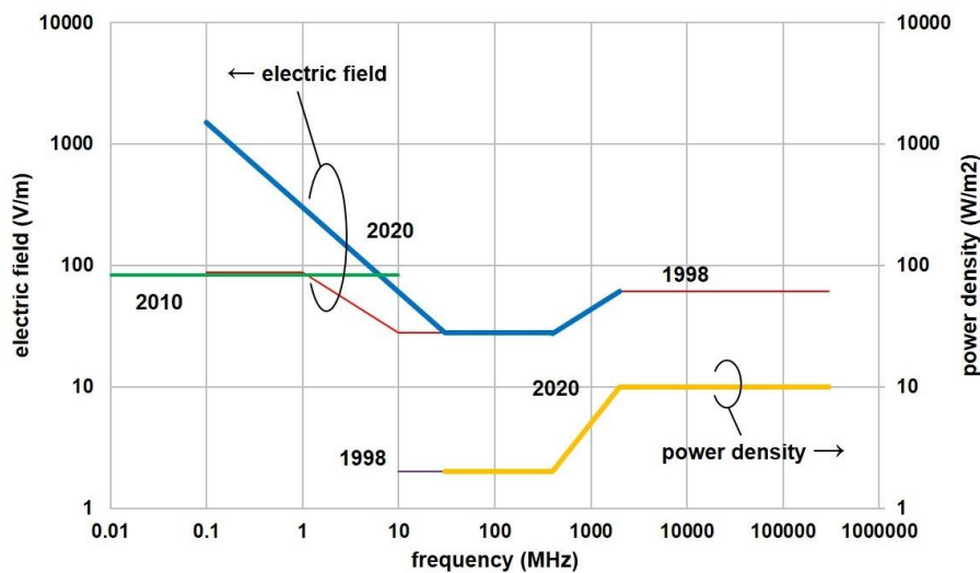
Figura 9 Niveles de referencia promedio de todo el cuerpo para el público en general (exposiciones > 30 min) para las directrices de la ICNIRP de 1998, 2010 (30 kHz a 10 MHz) y 2020, para la gama de frecuencias de 100 kHz a 300 GHz. Obsérvese que las unidades de los dos ejes verticales (campo eléctrico y densidad de potencia) son independientes entre sí [Fuente: ICNIRP].
